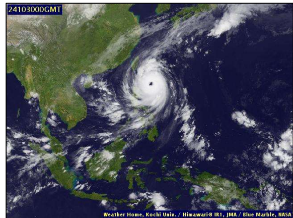
ภาพถ่ายดาวเทียม วันที่ ๓๐ ต.ค. ๒๕๖๗ เวลา ๐๗.๐๐ น.
