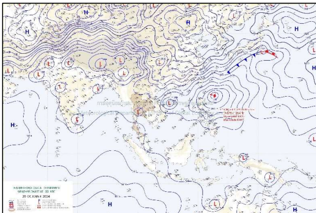
แผนที่อากาศ วันที่ ๓๐ ต.ค. ๒๕๖๗ เวลา ๐๑.๐๐ น.
